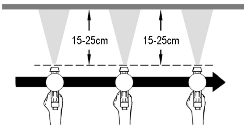
Správný způsob nanášení barvy.
